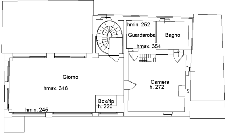
PIANO PRIMO
